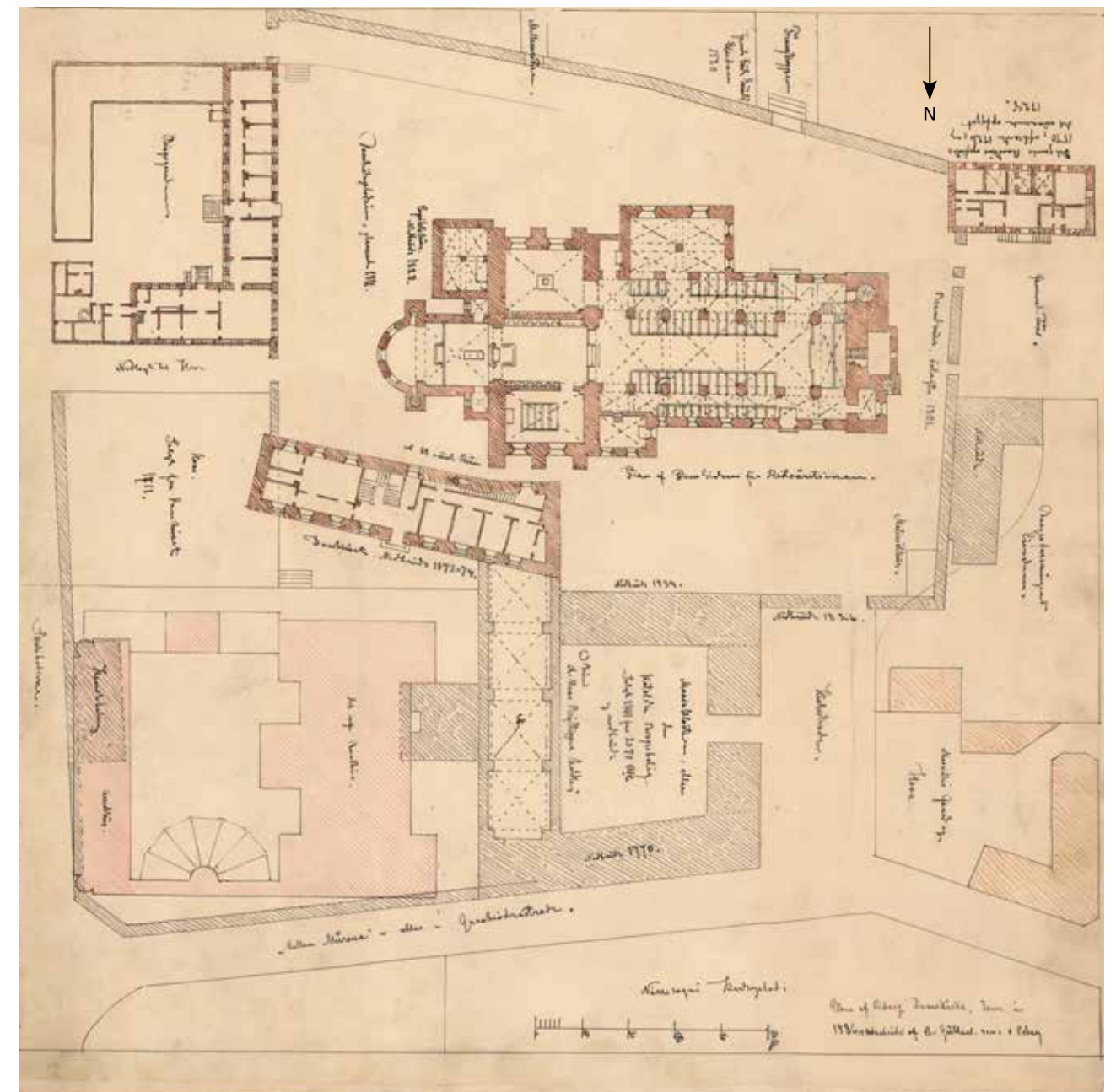
Figur 1.6. Viborg Domkirke med omgivelser – syd opad. Den store skråtliggende bygning nord for domkirken er Stænderhuset, der blev revet ned i 1873 for at give udsigt til den genopførte domkirke. Sammen med den anden store bygning mod nord med antydninger af hvælv, har huset udgjort hovedbygningen i den senmiddelalderlige bispegård. Den katolske bispegård var efterfølgeren af augustineres Maria Kloster, om end bygningerne muligvis ikke gik tilbage til klostertiden. Ikke alle detaljer på den meget store rekonstruktionstegning kan genfindes i dag. Rekonstruktion: Chr. Gullev 1886.
