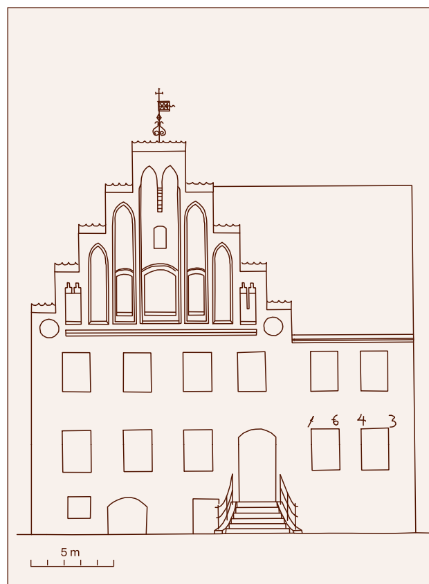
Figur 2.4. Opmåling af opstalten mod gaden for Sct. Mogens Gade nr. 9. Tegningen viser den planlagte gavltrekant. Grundlæggende svarer tegningen til husets nuværende udseende. Opmåling: H.C. Amberg før 1884, Viborg Museum, rentegning: Morten Larsen 2023.
